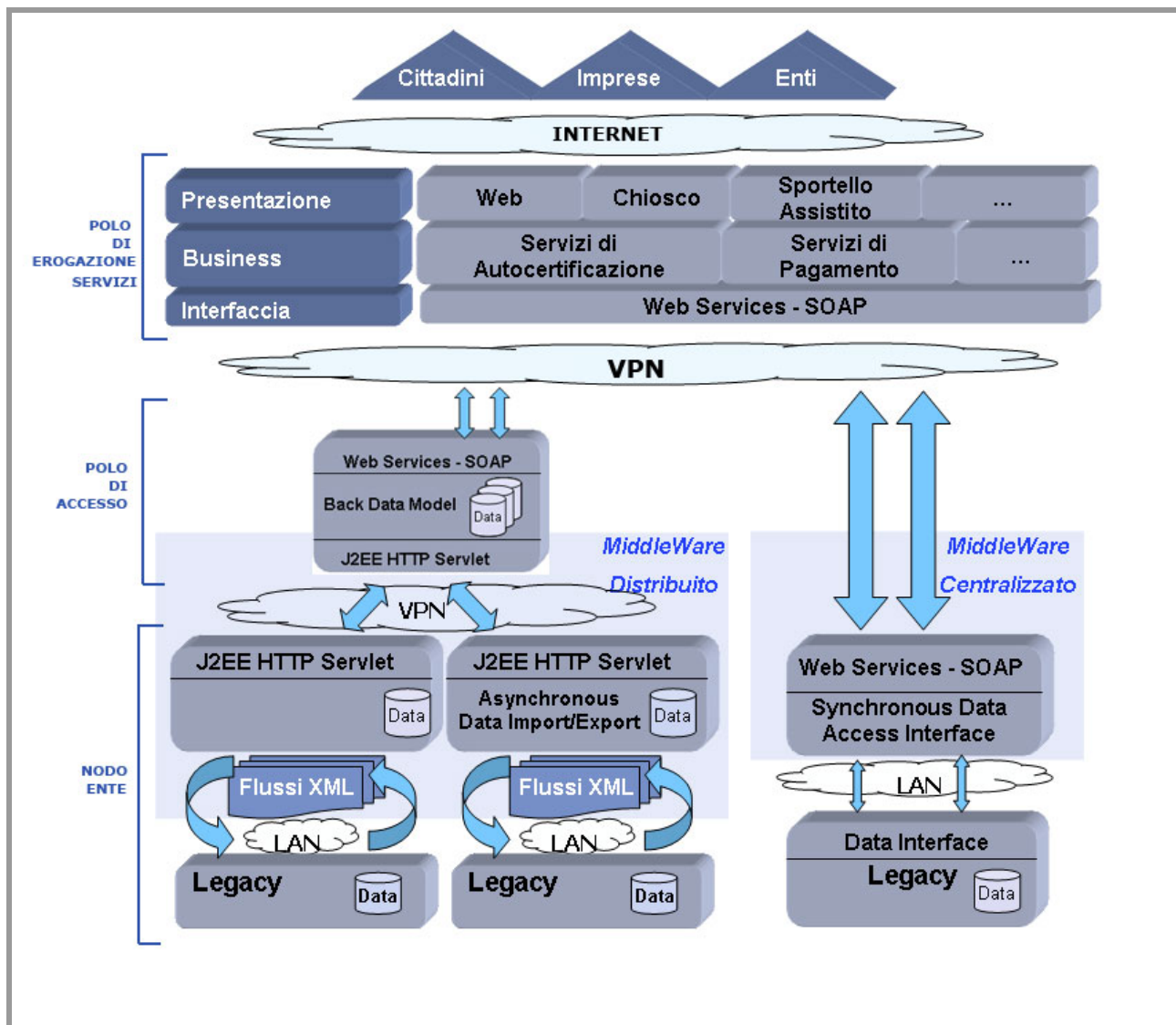
Fig. 1 – Architettura Tecnologica
